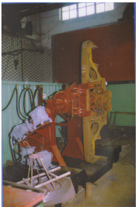
Кантувач для перевертання надресорних балок візка як при ремонті, так і при дефектоскопії дефектоскопом МД-17-П.
