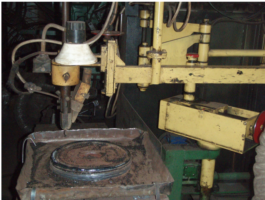
Кантувач для перевертання бокових рам візка
